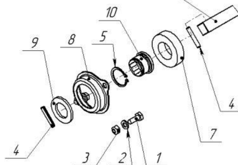
ОЗШ 01.614-вал зерновых и ОЗШ 01.611 туковых аппаратов
