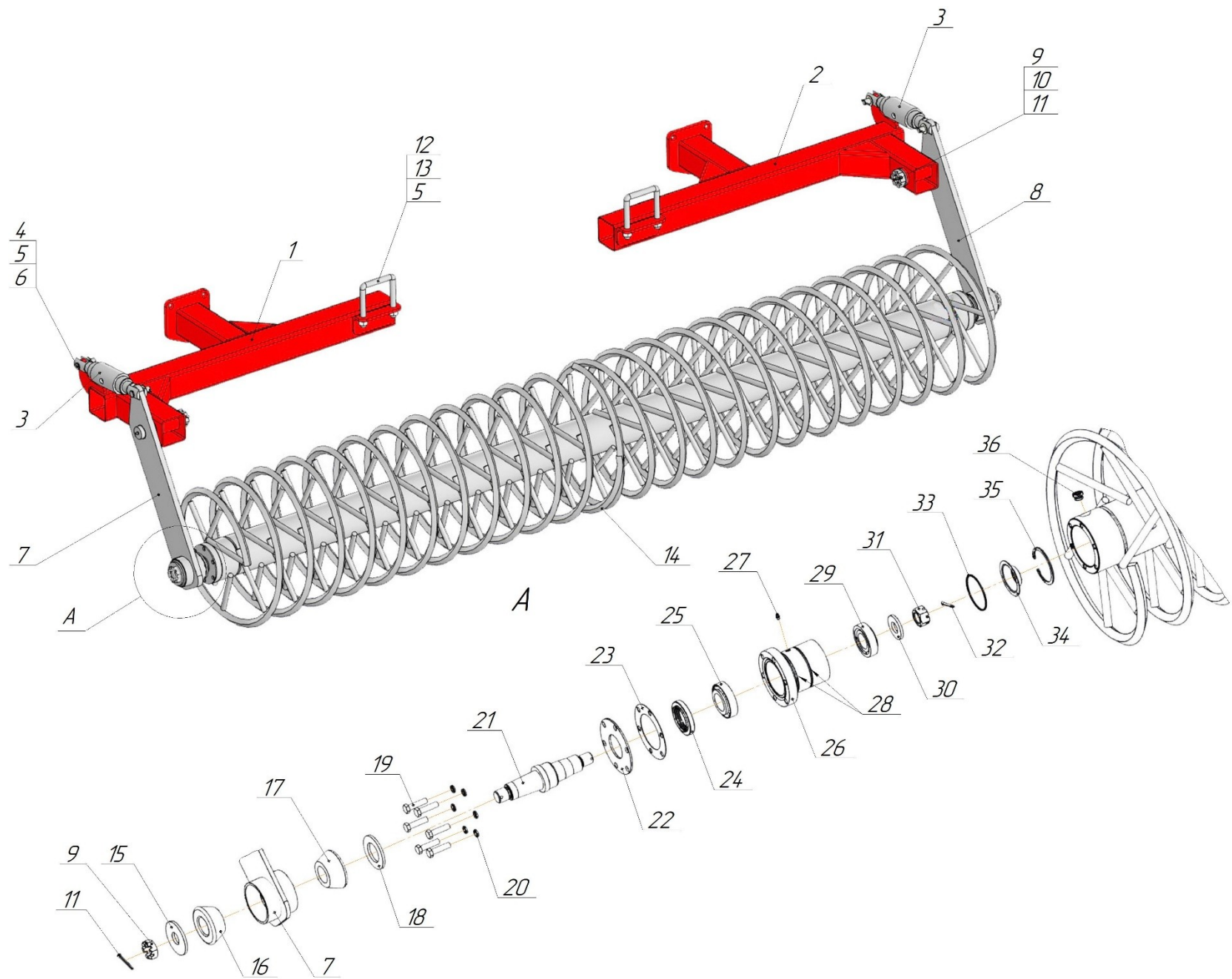
Рис. 5 – Шлейф-каток БДП 14.000-01 бороны дисковой прицепной БДП-3200-02/-06 (PALLADA 3200)
