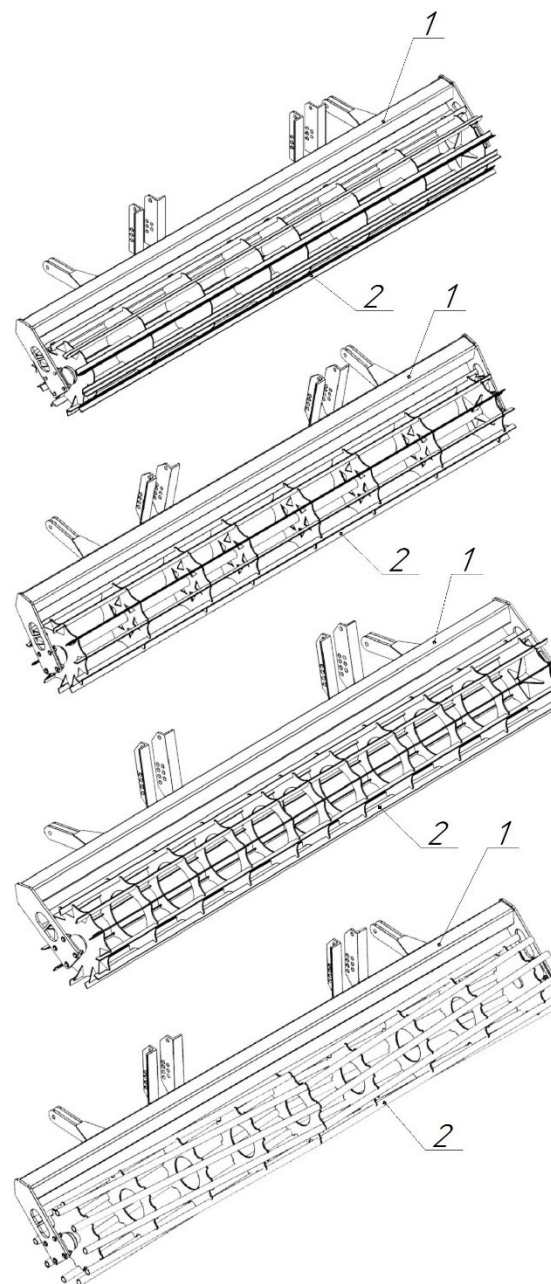
Рис. 4 – Каток прикатывающий бороны дисковой прицепной БДП-3200/-01/-03/-04/-05/-07/-08/-09 (PALLADA 3200)
