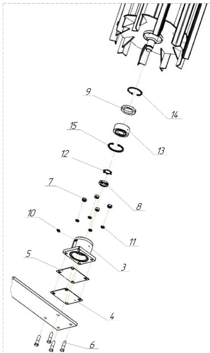
Рис. 4 – Каток прикатывающий бороны дисковой прицепной БДП-3200/-01/-03/-04/-05/-07/-08/-09 (PALLADA 3200)
