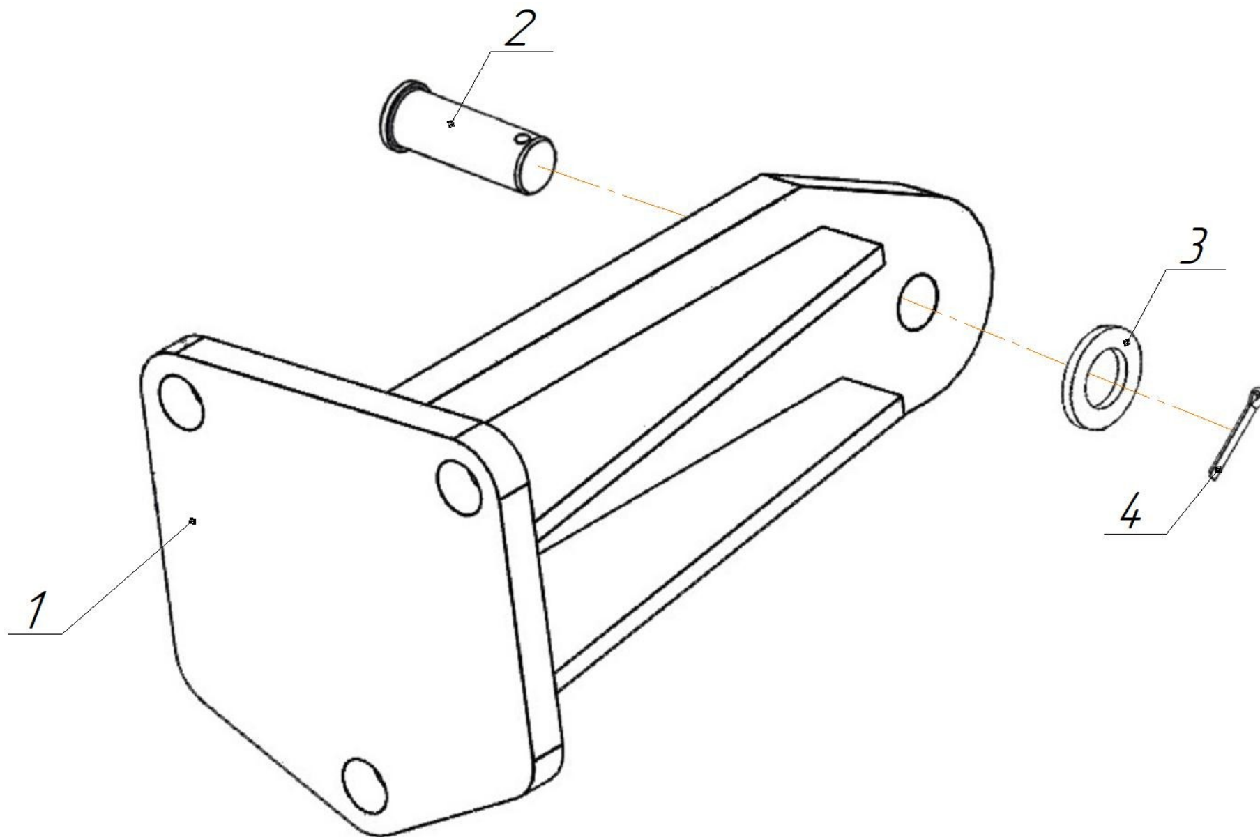
Рис. 8 – Кронштейн БДП 15.000 (-01) крепления катка прикатывающего для бороны дисковой прицепной БДП-3200/-01/-03/-04/-05/-07/-08/-09 (PALLADA 3200)
