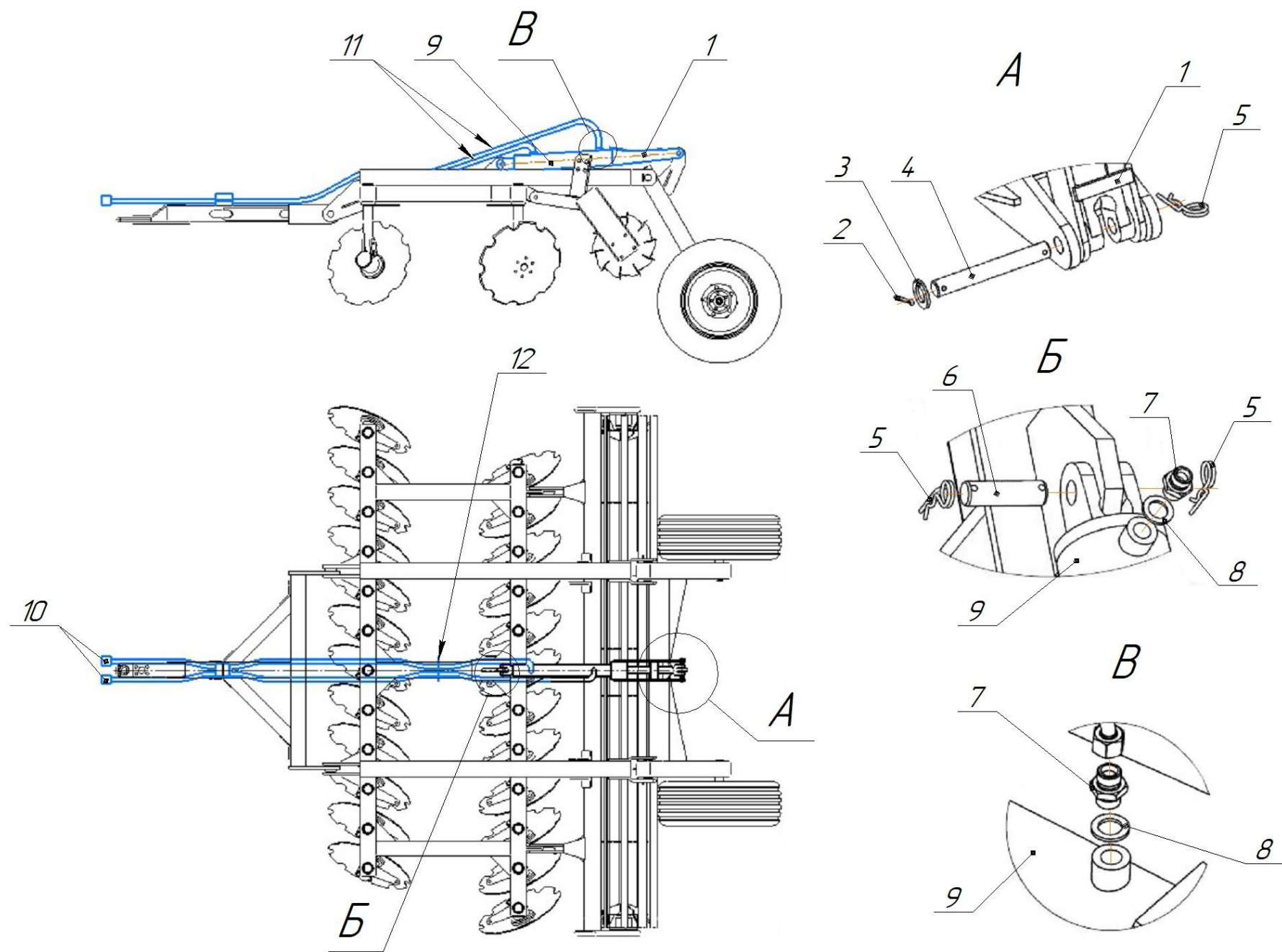
Рис. 11 – Гидротрасса БДП 07.000-01 для бороны дисковой прицепной БДП-3200 (PALLADA 3200)
