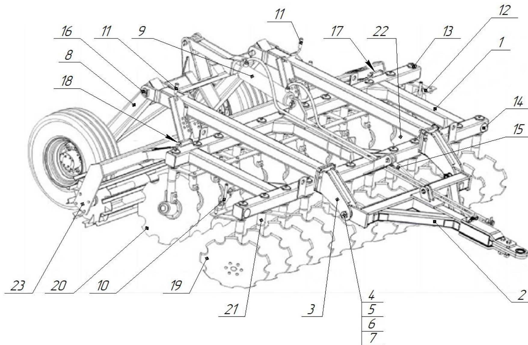
Рис. 1 – Общее устройство бороны дисковой прицепной БДП-3200 (PALLADA 3200)
